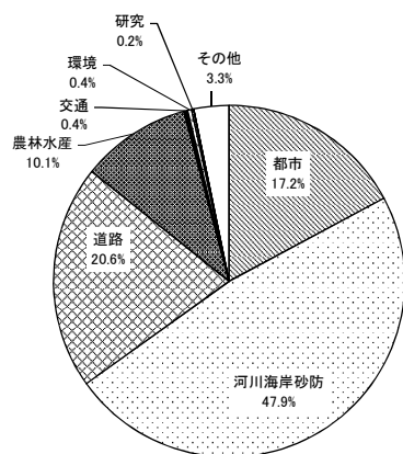
図-8-1 数値図化 測量目的別の内訳 ※表-1の数値図化、数値図化(同時調整含む)及び 既成図数値化の内訳
