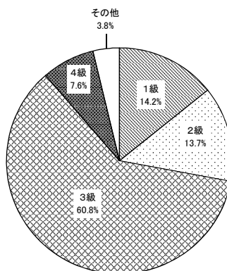
図-6-2 水準測量 等級別の内訳
