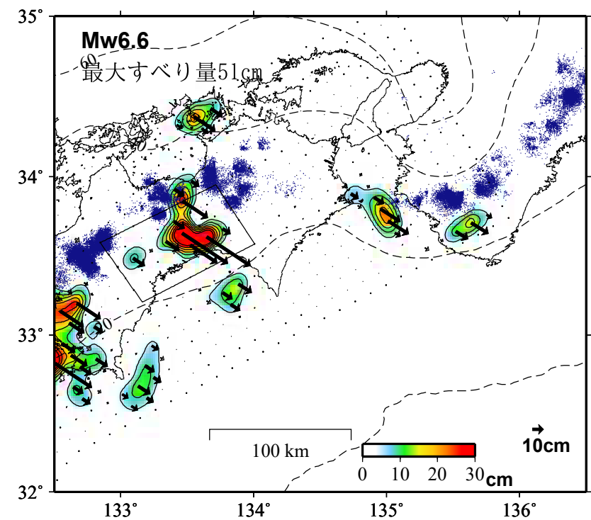
推定すべり分布 (2019-01-01/2024-05-12)
