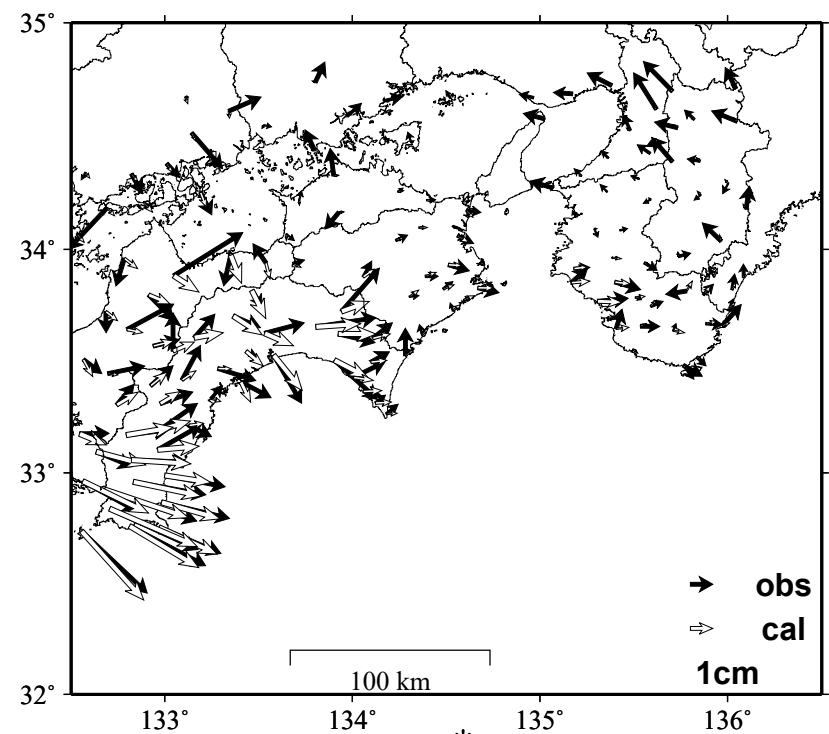
観測値（黒）と計算値（白）の比較 (2019-01-01/2024-05-12)
