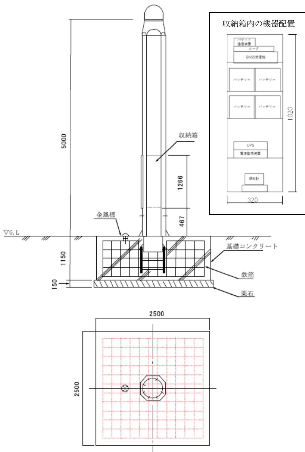
電子基準点構造図
