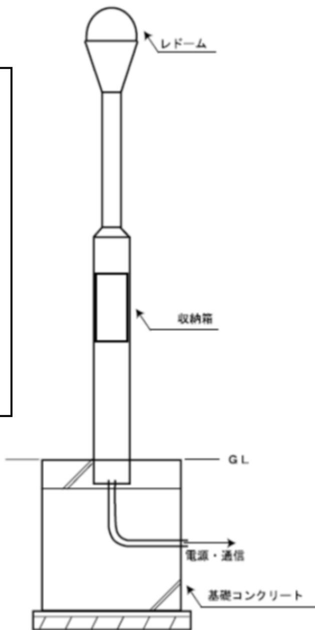
電子基準点構造図
