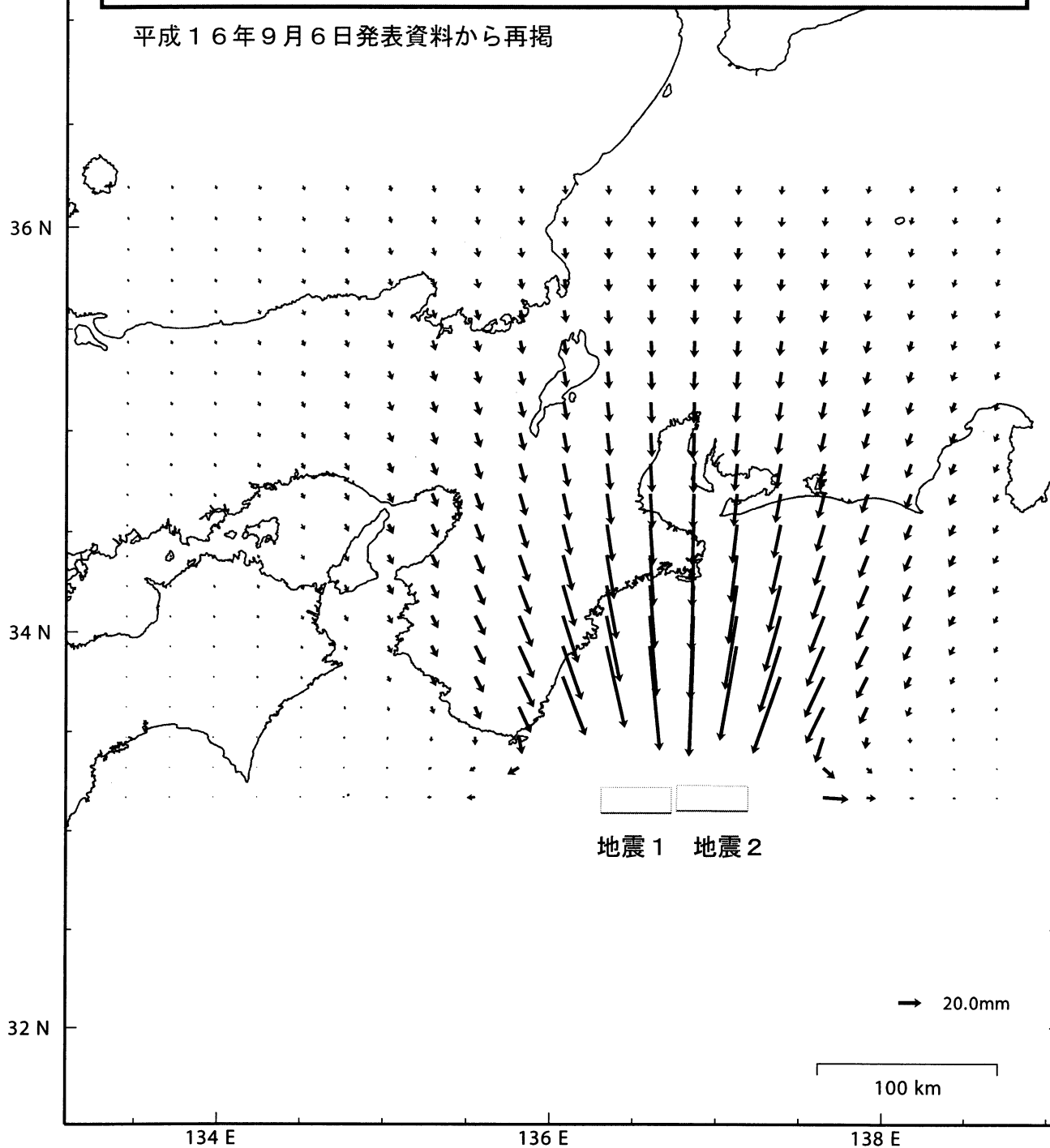
断層モデル
