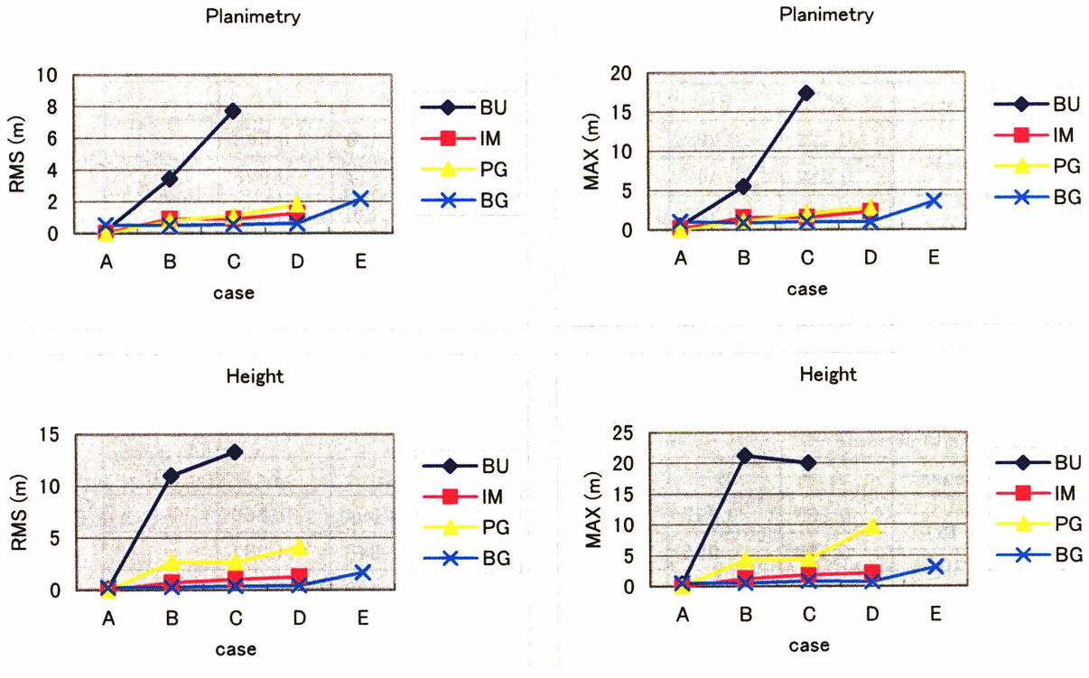
図-1 各種空中三角測量手法の比較実験結果 (伊豆大島地区)
