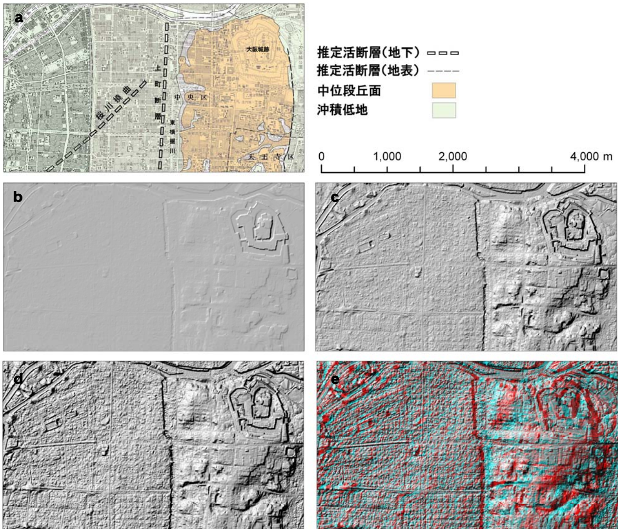
図-5 (a) 都市圏活断層図「大阪東北部(中田ほか, 2009)」「大阪西北部(中田ほか, 1996)」の一部。中位段丘が上町台地。推定活断層(地下)として上町断層, 桜川撓曲がある。(b~d) 航空レーザ測量5mDEMから作成した陰影図。Z=1倍(b), Z=10倍(c), 標高値の対数を定数倍して作成(d)。(e)は(d)及びその元になった高さデータから作成した余色立体図。
