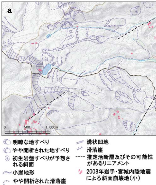
図-9 (a) 岩手・宮城内陸地震詳細活断層図(国土地理院, 2009)の一部。(b) 航空レーザ測量0.2秒(約5m)メッシュDEMから作成した余色立体図(Z=5).
