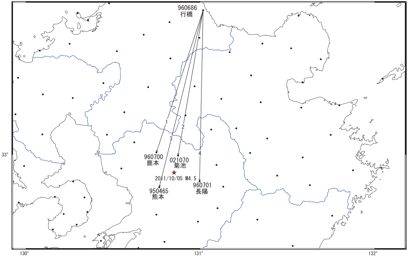
基線図
