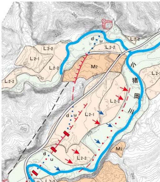
図-7 楓木立の活断層分布（裏面解説の図の一部） 活断層は赤線、推定活断層は黒の破線、活撓曲は赤矢印、傾動は青矢印
