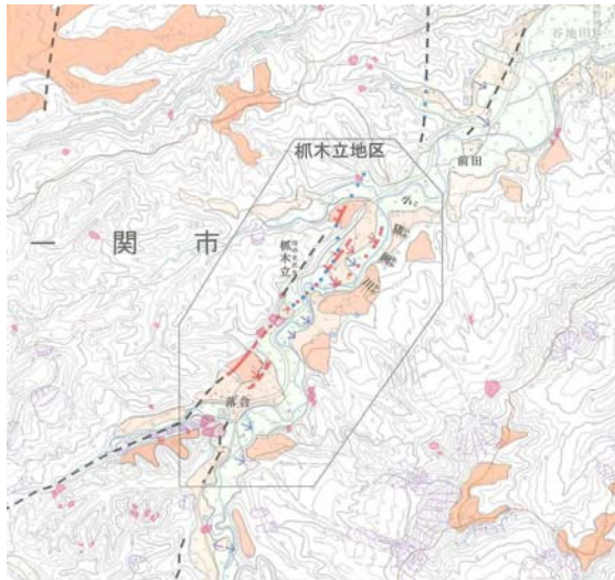
図-6 楓木立付近の活断層の変位地形（詳細活断層図、活断層は赤線、推定活断層は黒の破線、活撓曲は赤矢印、傾動は青矢印）
