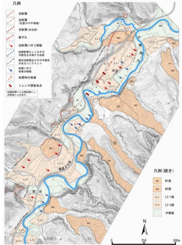
図-2 爪木立地区 (活断層及び地形区分図)
