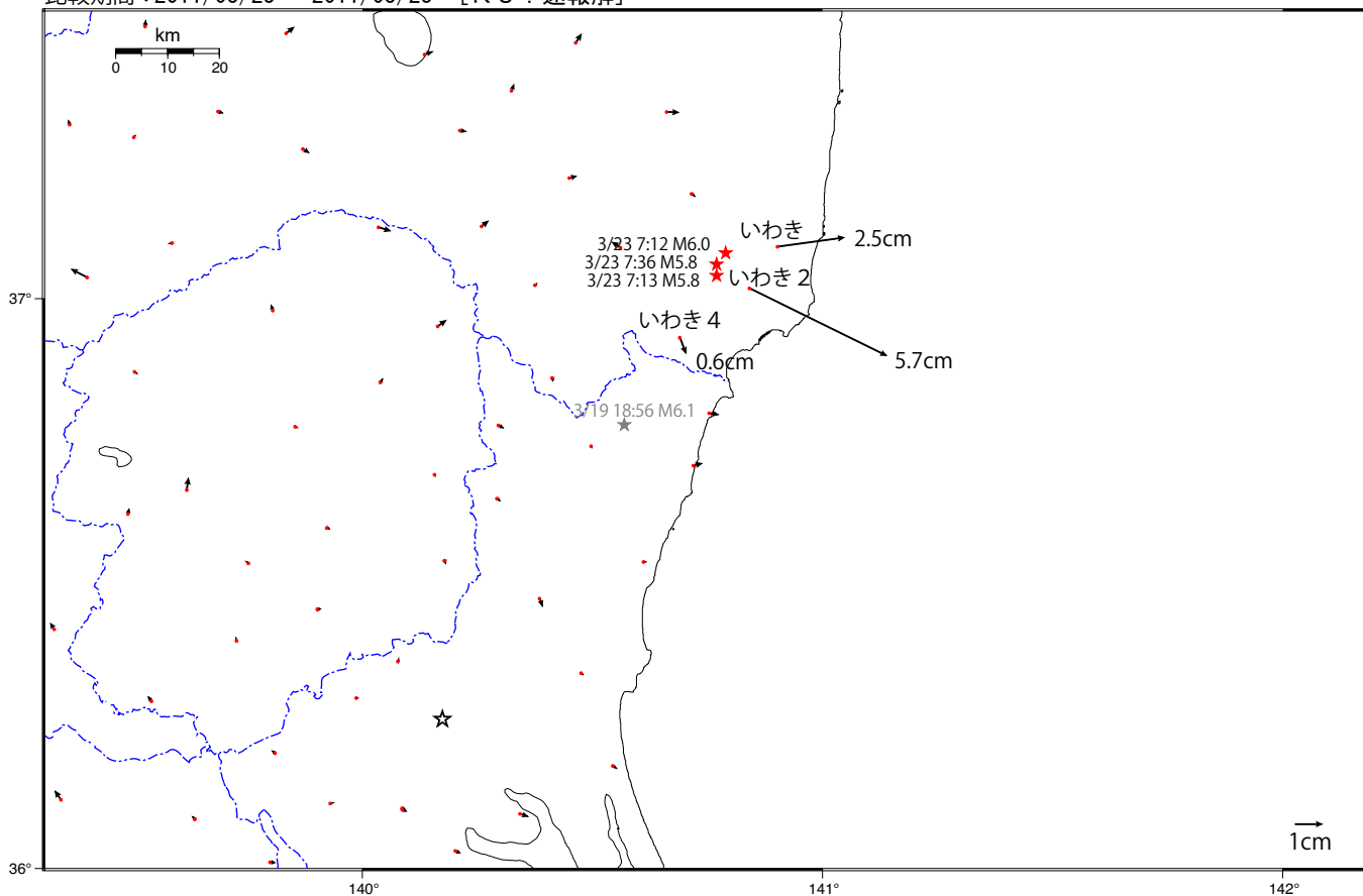
変動ベクトル図(水平)
