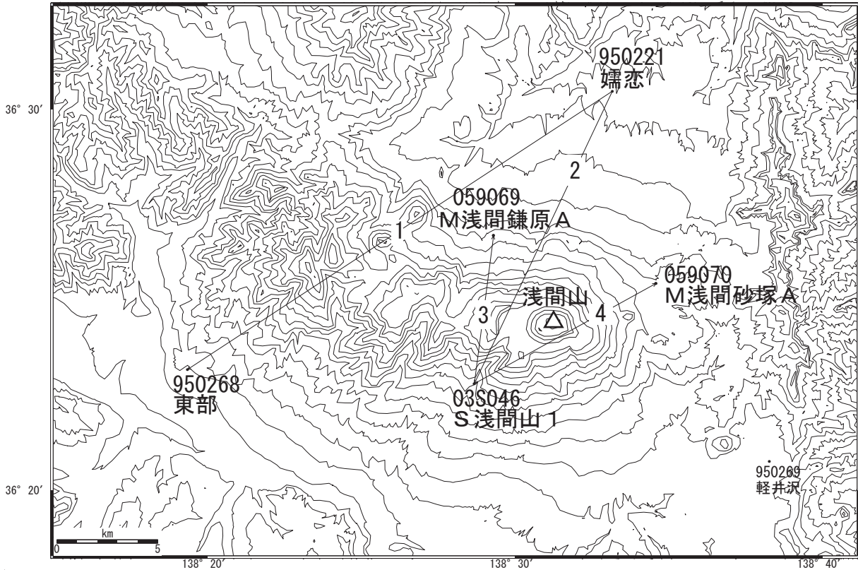
浅間山周辺 GPS連続観測基線図
