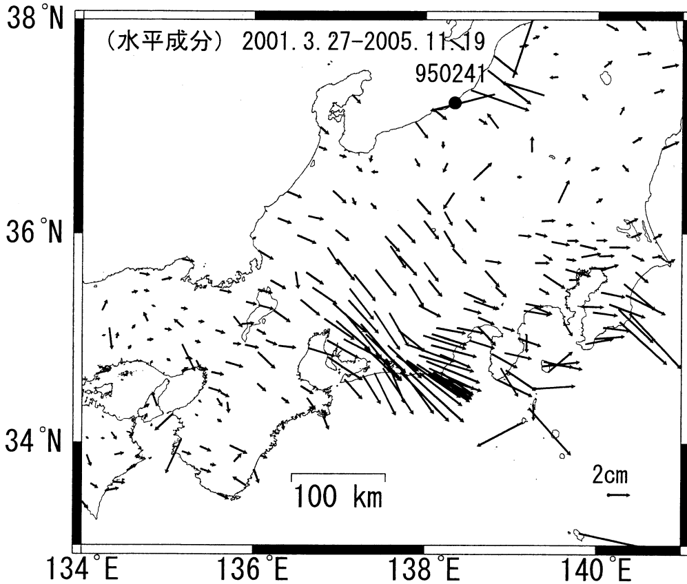
定常的な地殻変動
