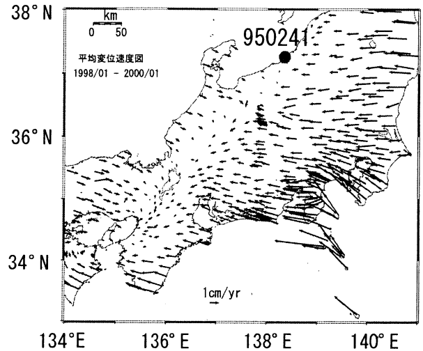
定常的な地殻変動
