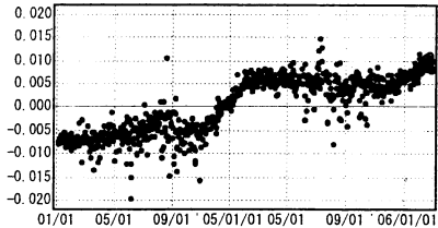
(m) (2) 鹿児島3 (960721)→桜島(960719) 斜距離
