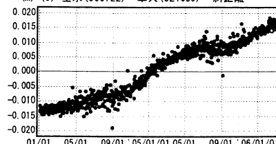
(m) (9) 垂水(960722)→隼人(021089) 斜距離
