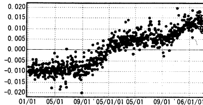
(m) (5) 鹿児島福山(950489)→隼人(021089) 斜距離
