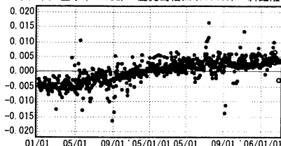
(m) (6) 垂水(960722)→鹿児島福山(950489) 斜距離
