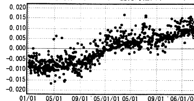
(m) (8) 鹿児島郡山(960776)→鹿児島福山(950489) 斜距離
