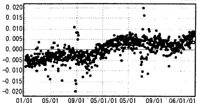
(m) (3) 鹿児島3 (960721)→鹿児島2 (960720) 斜距離
