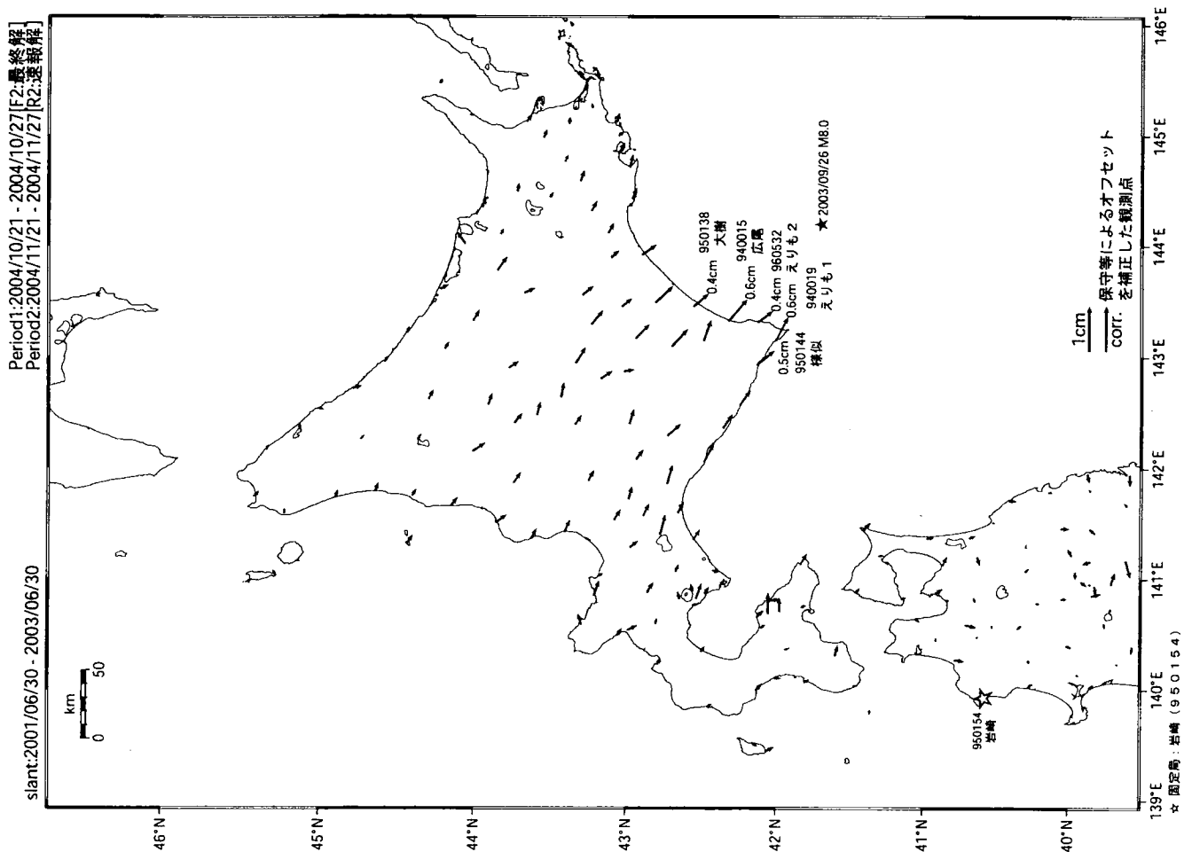
平成15年(2003年)十勝沖地震後の水平変動(傾斜・年周・半年周補正)
