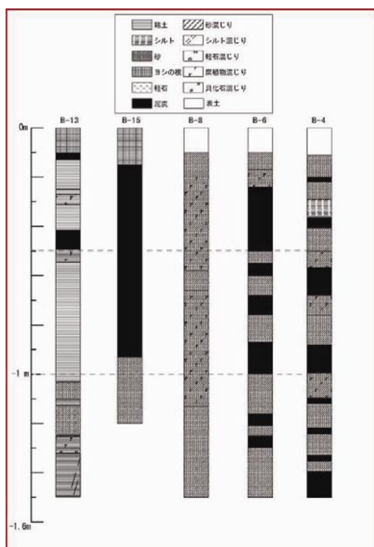
図-9 簡易ボーリング柱状図
