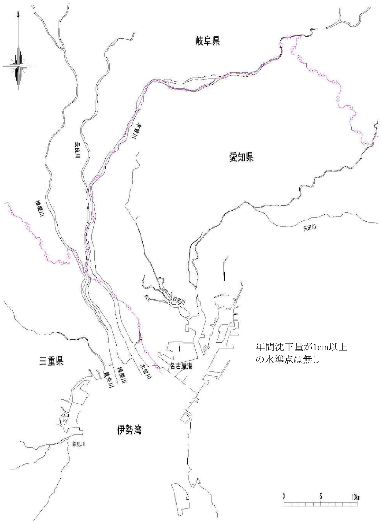
図-2 令和4年度における年間沈下量1cm 以上の水準点位置
