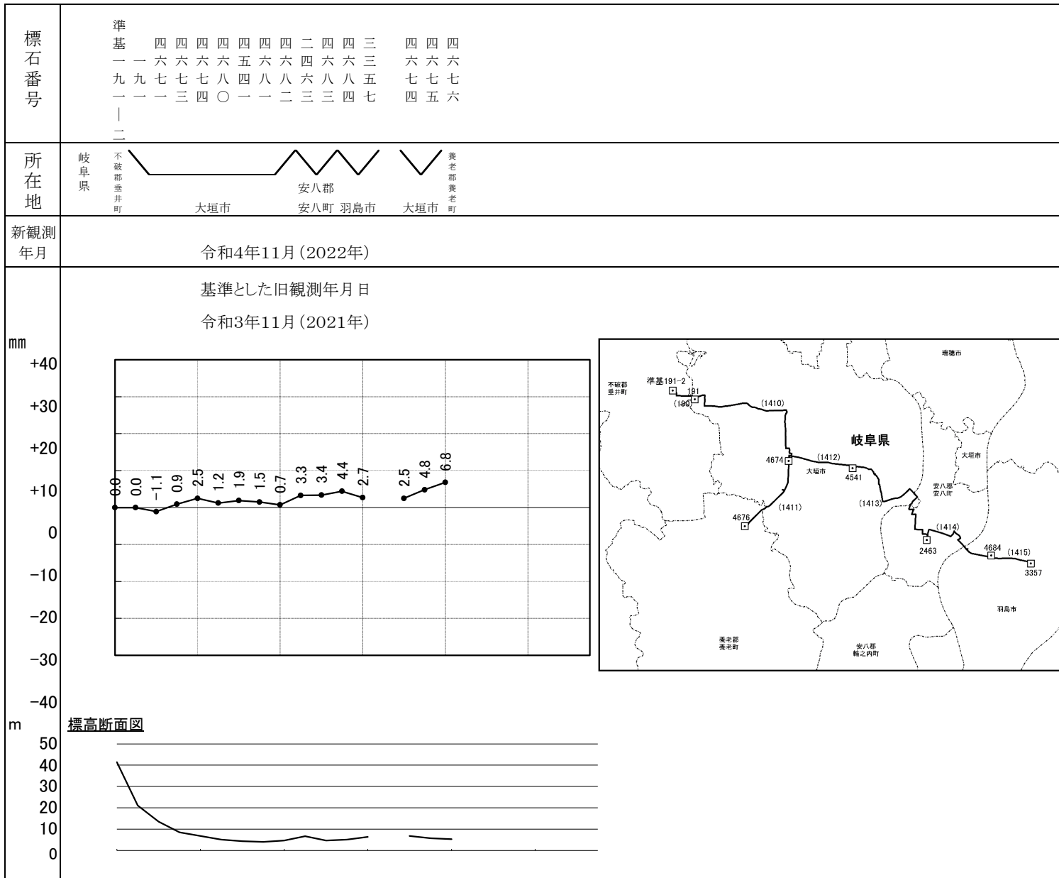
図5 - 3 基本水準点変動図
