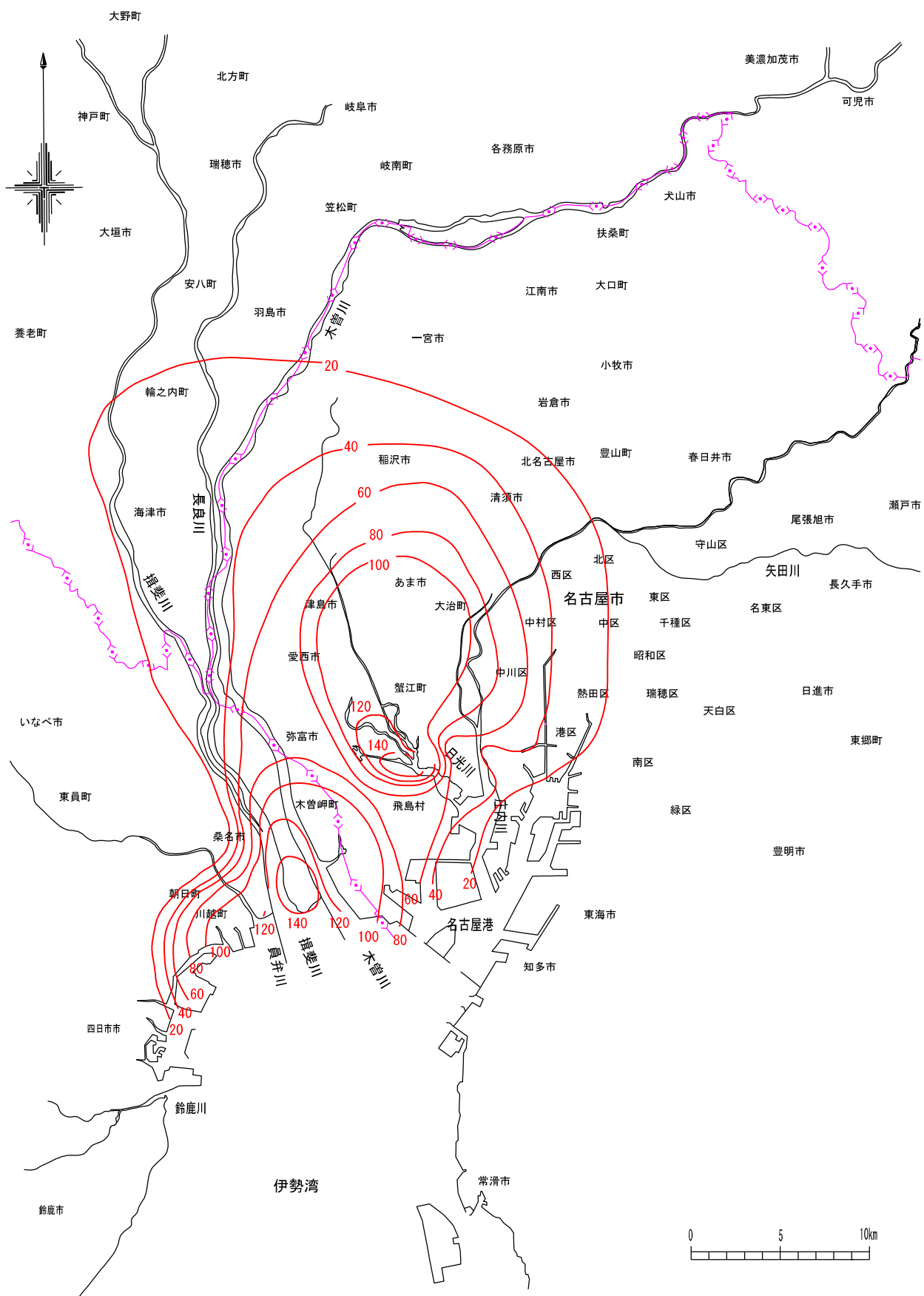
図-3 昭和36年以降の累積沈下量等量線図(単位:cm) (昭和36年2月～令和4年11月)
