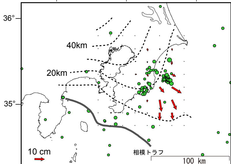
B ゆっくり滑りの発生した期間: 2002年 10月4日～10月14日頃 解析に使用したGPSデータの期間: 2002年 9月1日～12月2日 最大滑り量 約13cm Mw 6.5
