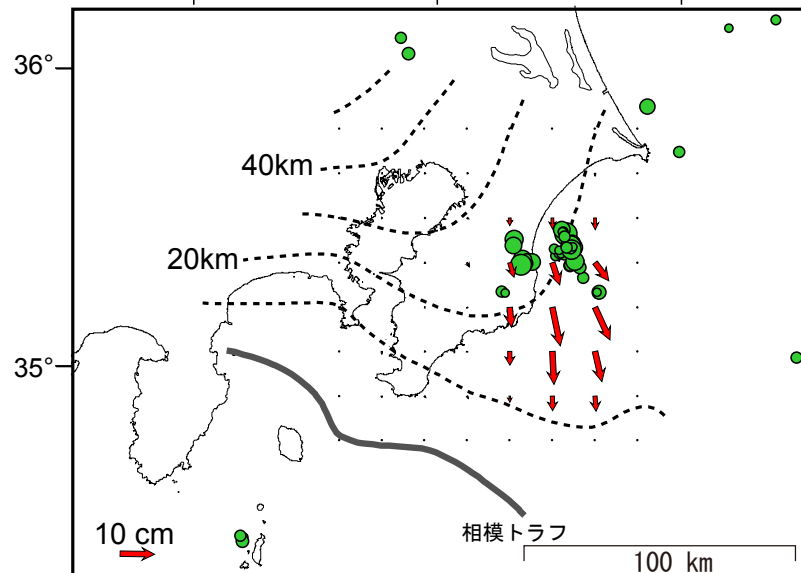
C ゆっくり滑りの発生した期間: 2007年 8月13日～8月23日頃 解析に使用したGPSデータの期間: 2007年 8月1日～8月26日 最大滑り量 約12cm Mw 6.6
