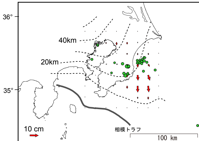
A ゆっくり滑りの発生した期間: 1996年 5月14日～5月24日頃 解析に使用したGPSデータの期間: 1996年 4月8日～6月10日 最大滑り量 約8cm Mw 6.4
