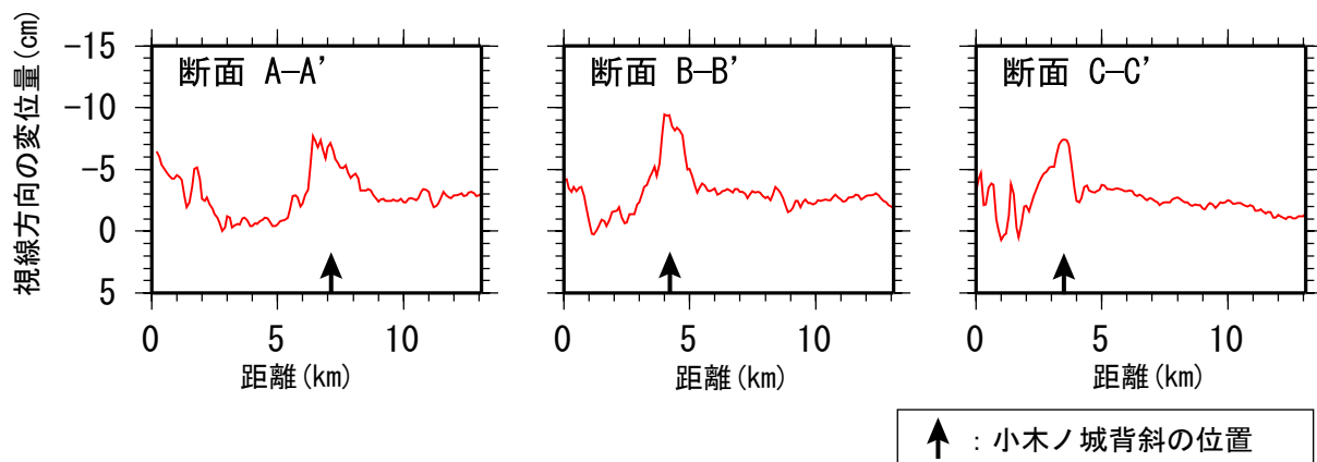
带状隆起の断面図
